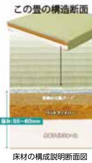
床材の構成説明断面図
